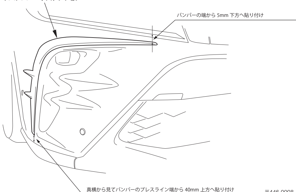
フロントバンパーエクステンション
