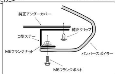
〈図3〉断面図
