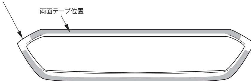
フロントグリルエクステンション(裏側)
